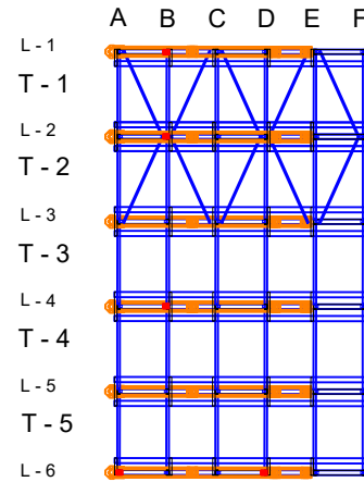
BLOQUE 1 ESTRUCTURA DRIVEIN TIPO STOR 60 POSICIONES
