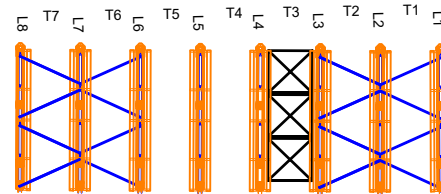
DRIVE IN MEXROLL BLOQUE 4 63 posiciones
